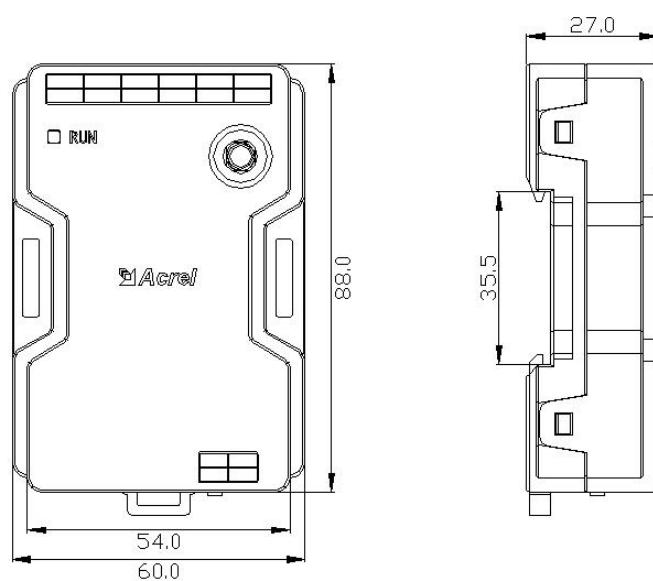
ATE300M
