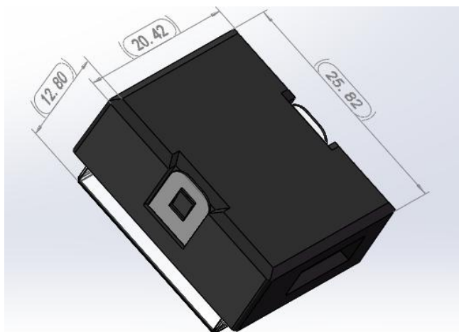
ATE400
